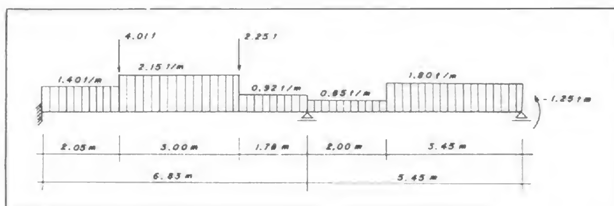
Figura 3 — Viga -- exemplo.
